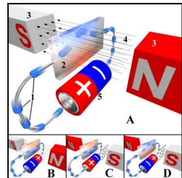
Schematische werking van een Hall-Sensor
